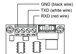
SA-232 wiring
